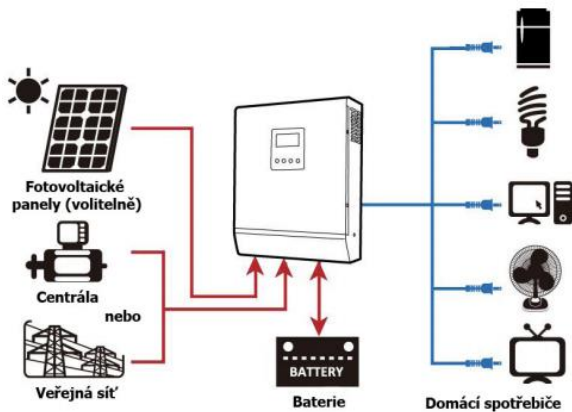
Obrázek 1: hybridní systém
